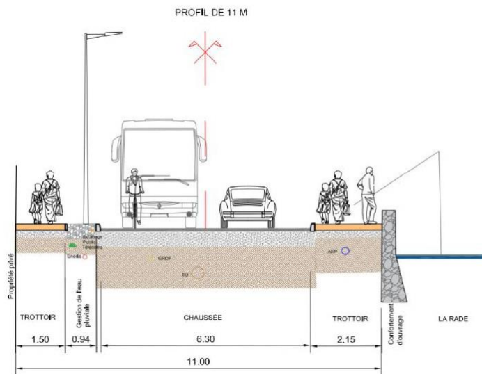
Profil de la corniche mesurant 11m / aménagement actuel
